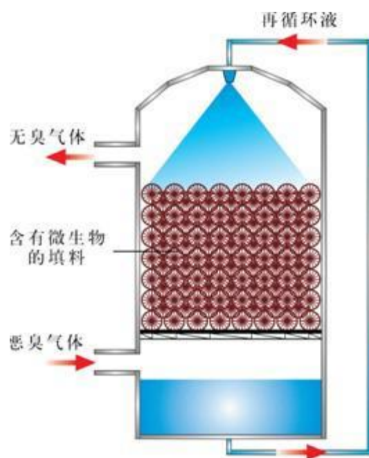
图7-1 生物除臭装置图
