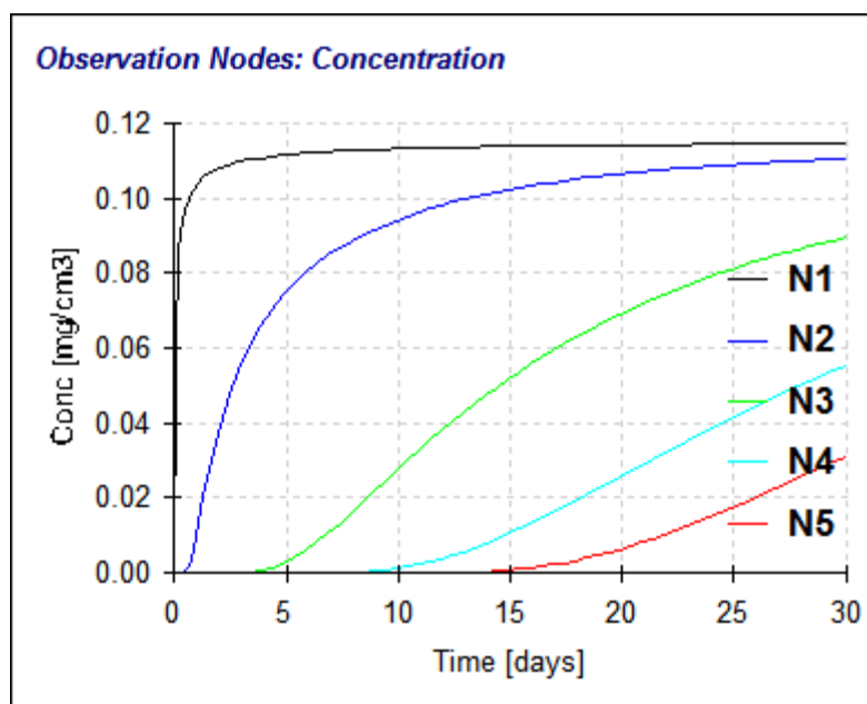
图5-12 不同深度处 COD 污染物浓度随时间变化曲线
