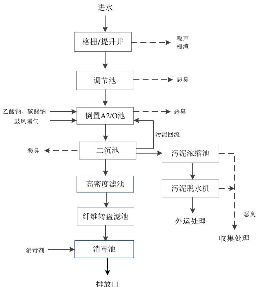
图3-1 污水处理工艺流程及产污环节图
